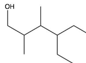
4-éthyl-2,3-diméthylhexan-1-ol
