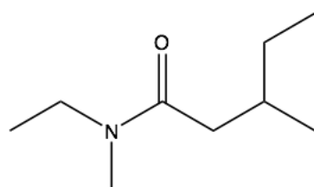
N-éthyl-N-méthyl-3-méthylpentanamide
