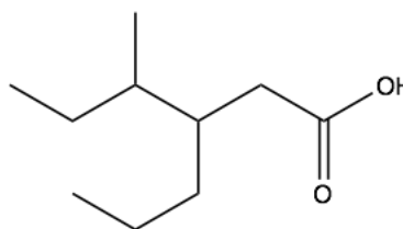
acide 4-méthyl-3-propylhexanoïque
