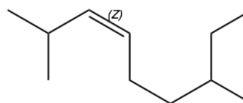
(Z)-2,7-diméthylnon-3-ène
