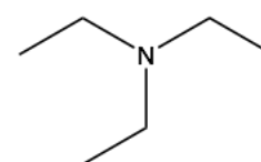
N,N-diéthyl-éthanamine
