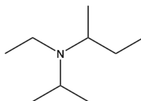
N-éthyl-N-(méthyléthyl)-butan-2-amine
