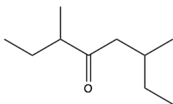
3,6-diméthyl-octan-4-one
