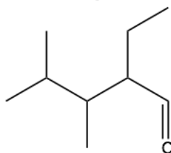
2-éthyl-3,4-diméthylpentanal
