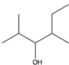
2,4-diméthylhexan-3-ol
